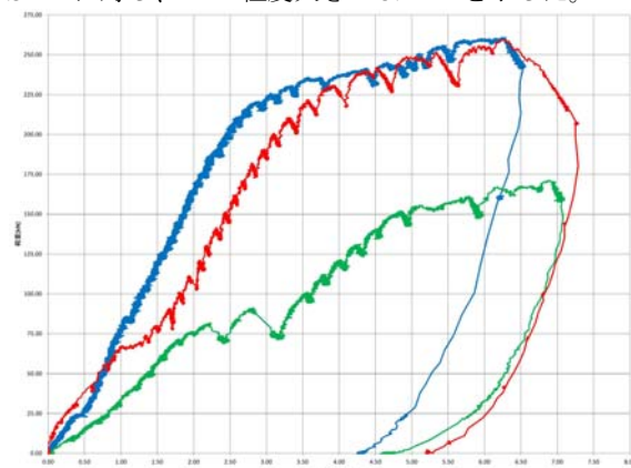
図-3 荷重-変位図
