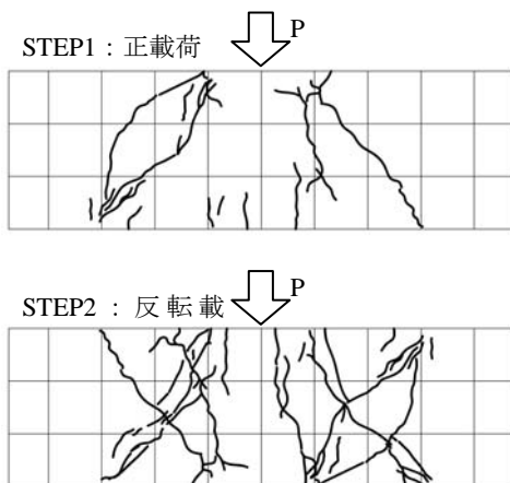
図-2 供試体クラック図
